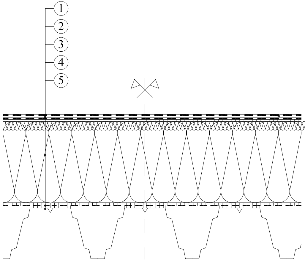
Ragasztásos rögzítés
