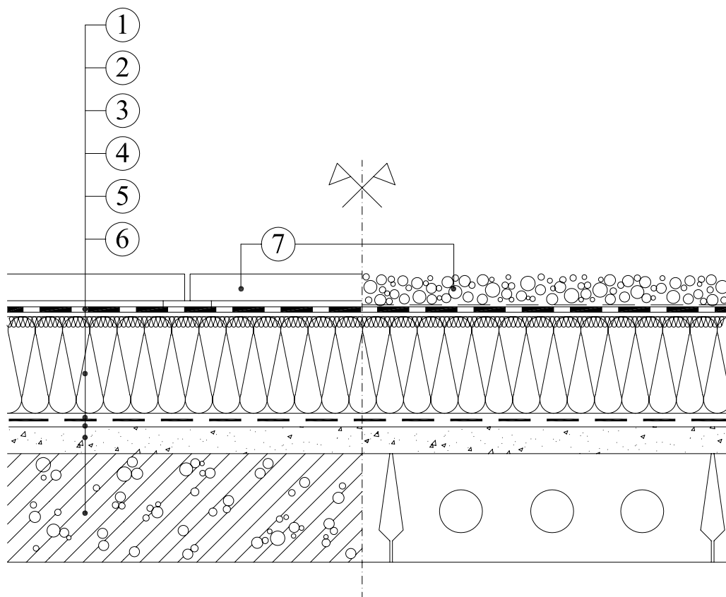
Leterheléses rögzítés beton lapokkal
