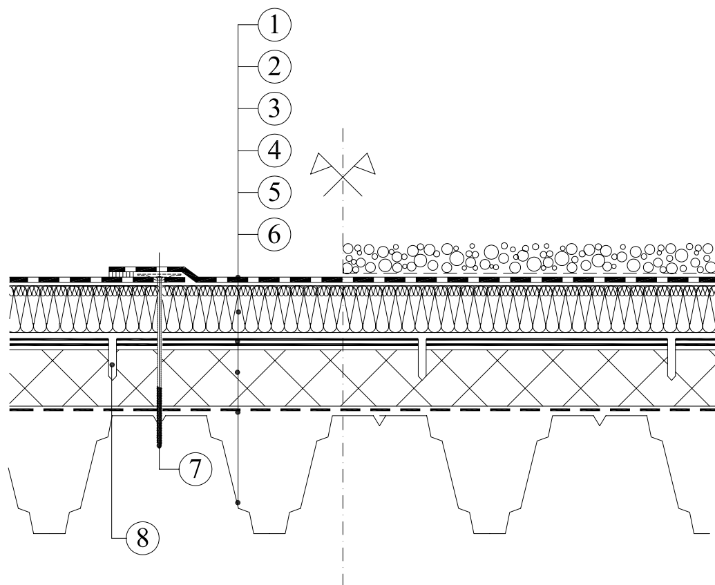
Mechanikai rögzítés
