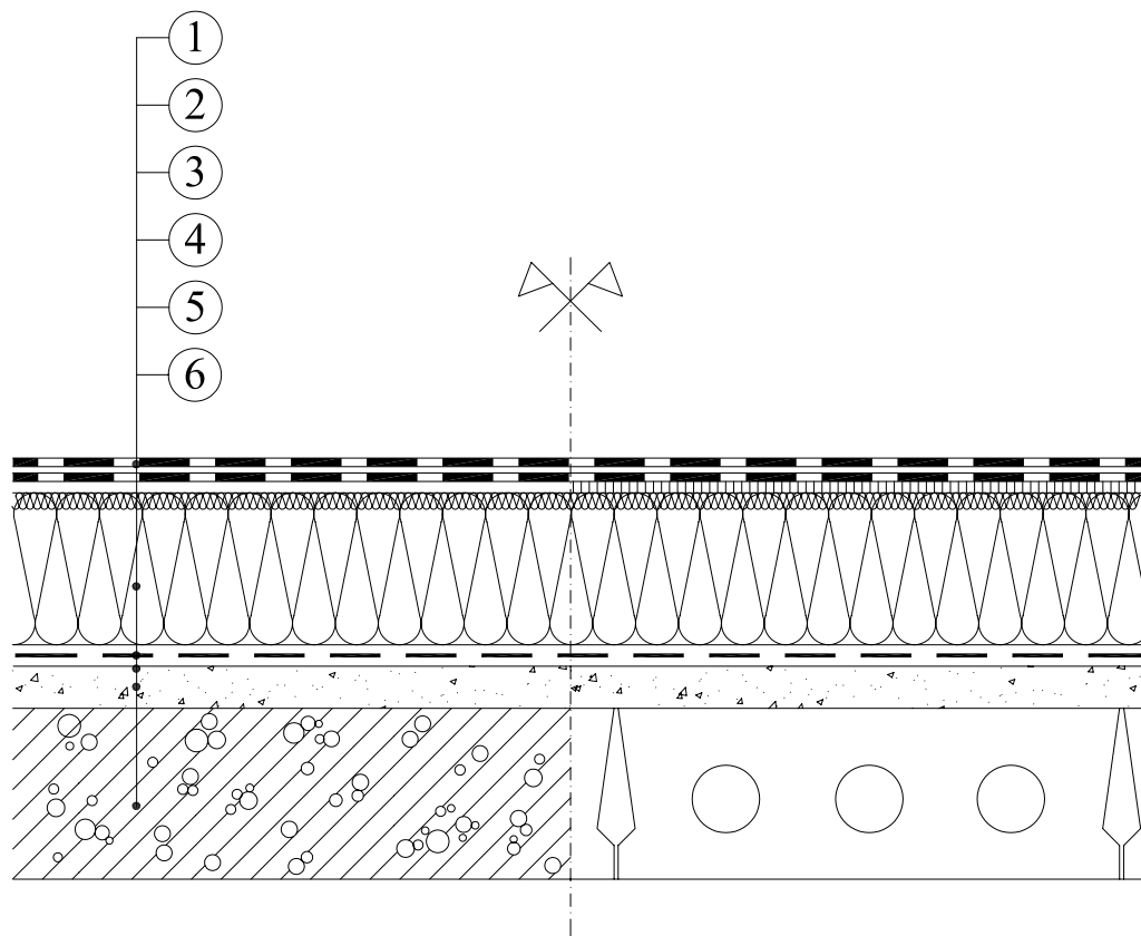
Hegesztett rögzítés
